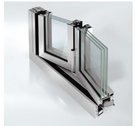
Schüco AS FD 90.HI (umlaufender Blendrahmen, nach innen oder außen öffnend) Schüco AS FD 90.HI (continuous outer frame, inward or outward-opening)
